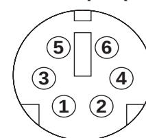
Mini Din 6-pin (Male)
