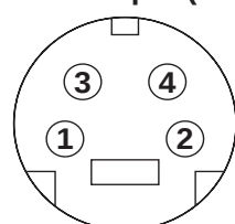
Mini Din 4-pin (Male)
