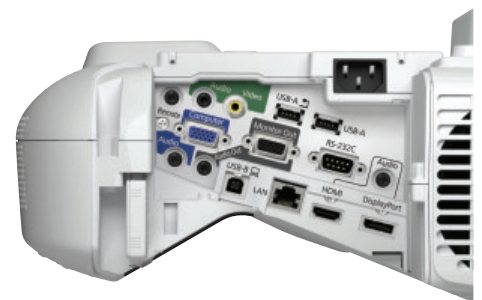
EB-1410Wi / EB-1400Wi interface
